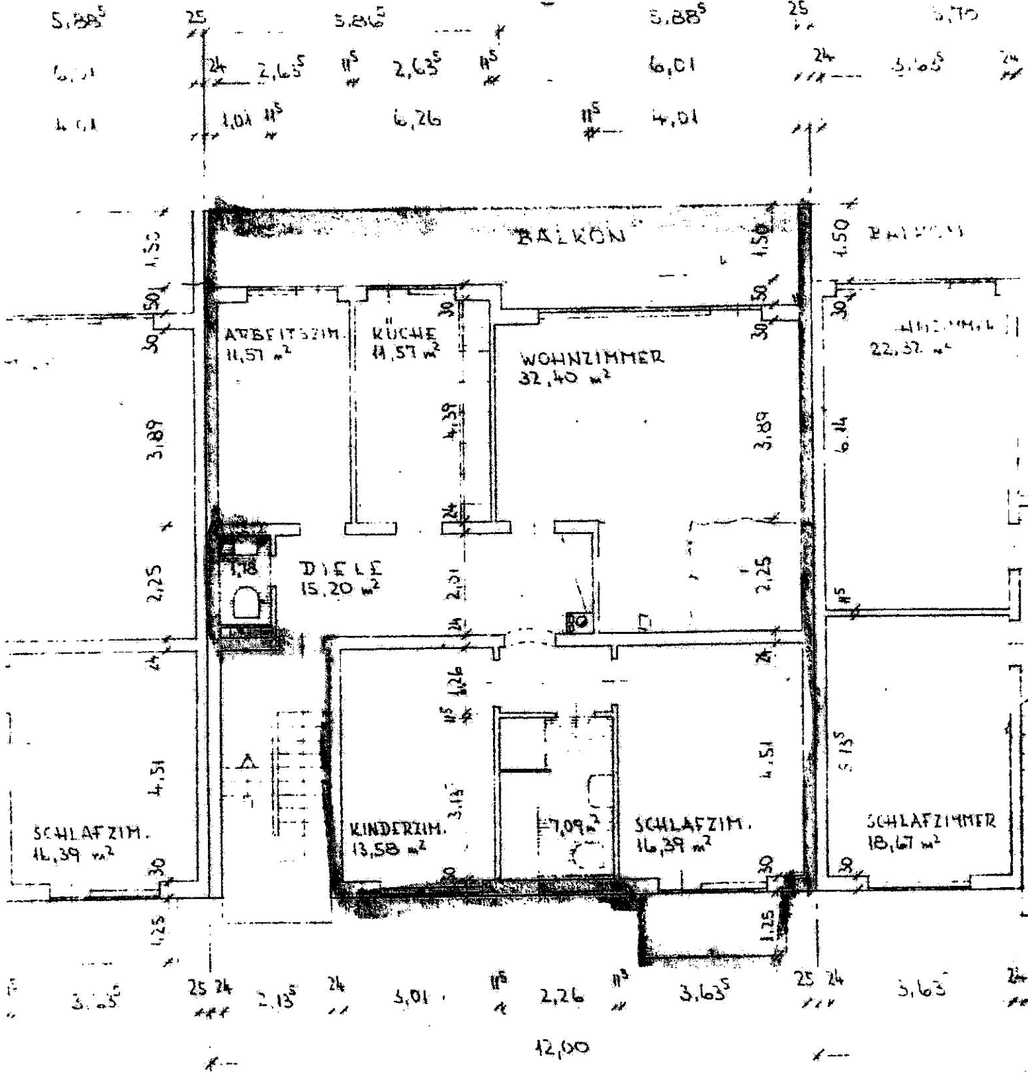
Erdgeschoß - 2. Obergeschoß
